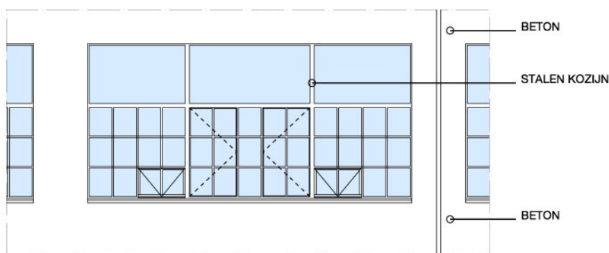
Buitenaanzicht gevel met kozijnindeling
