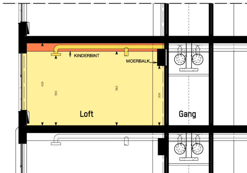
Doorsnede
