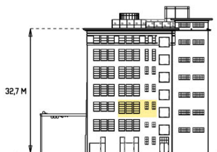
Westgevel
