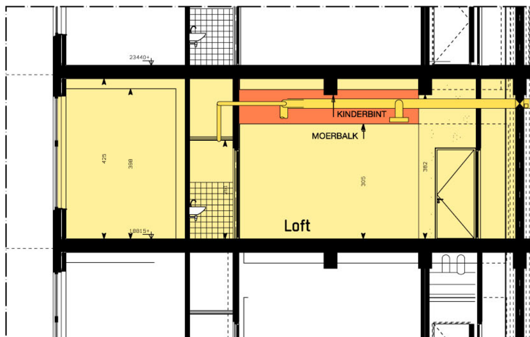
Doorsnede
