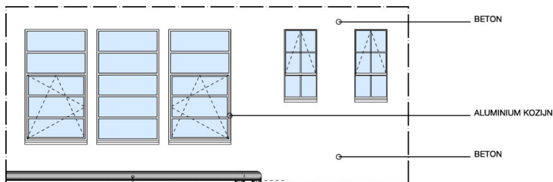
Buitenaanzicht gevel met kozijnindeling
