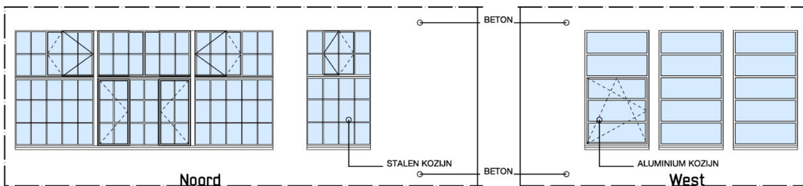
Buitenaanzicht gevel met kozijnindeling
